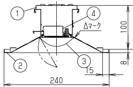
断面詳細図
