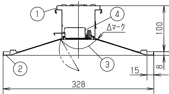
断面詳細図
