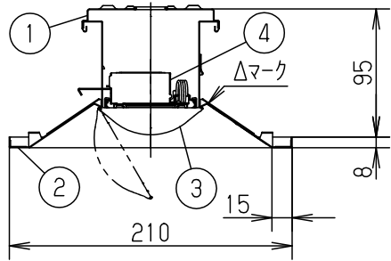
断面詳細図
